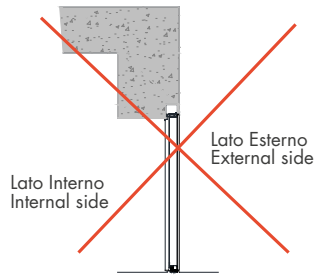
Installazione non corretta della porta Incorrect door installation
