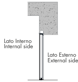
Installazione corretta della porta Correct door installation
